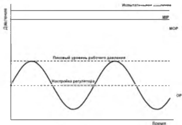
Рисунок 1 – Соотношение давлений
